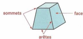
Sur ce dessin, on ne voit pas toutes les faces du polyèdre et certaines faces sont déformées.
